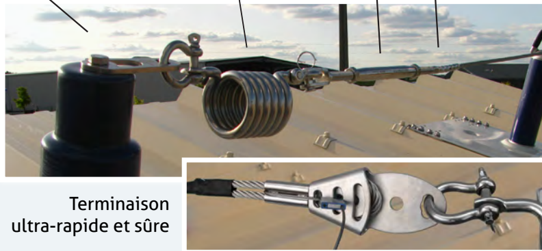
Poteau de départ Absorbeur avec témoin de chute Tendeur Cable
